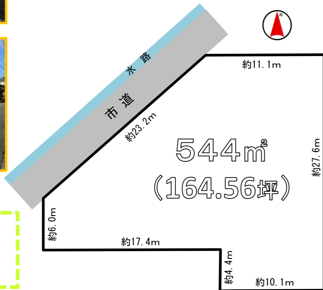
土地概略図
